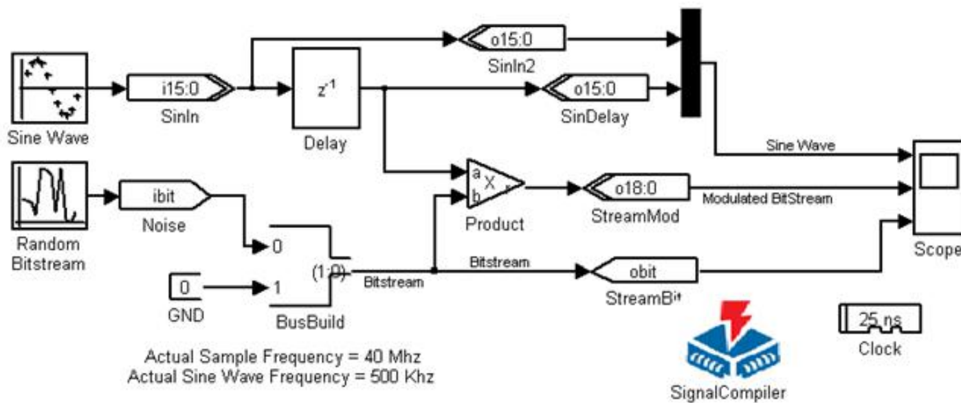
图 11-63 正弦调制信号模型
