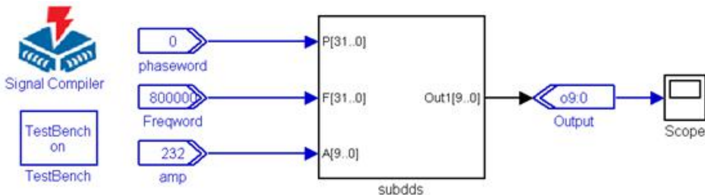
图 11-44 DDS 系统
