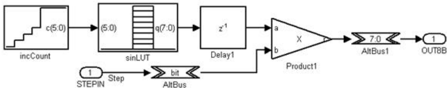
图 11-40 更改了端口和端口名的子系统图
