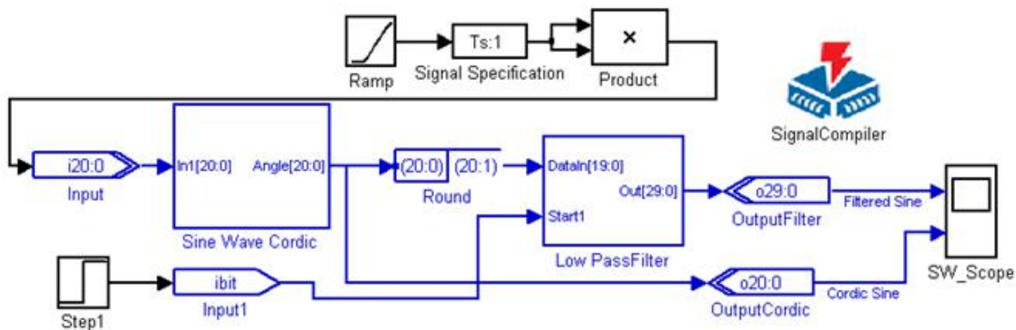
图 11-68 扫频滤波信号发生器模型 FreqSweep.mdl
