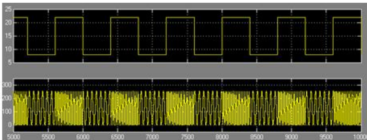
图 11-56 FSK 发生器 Simulink (软件) 仿真波形
