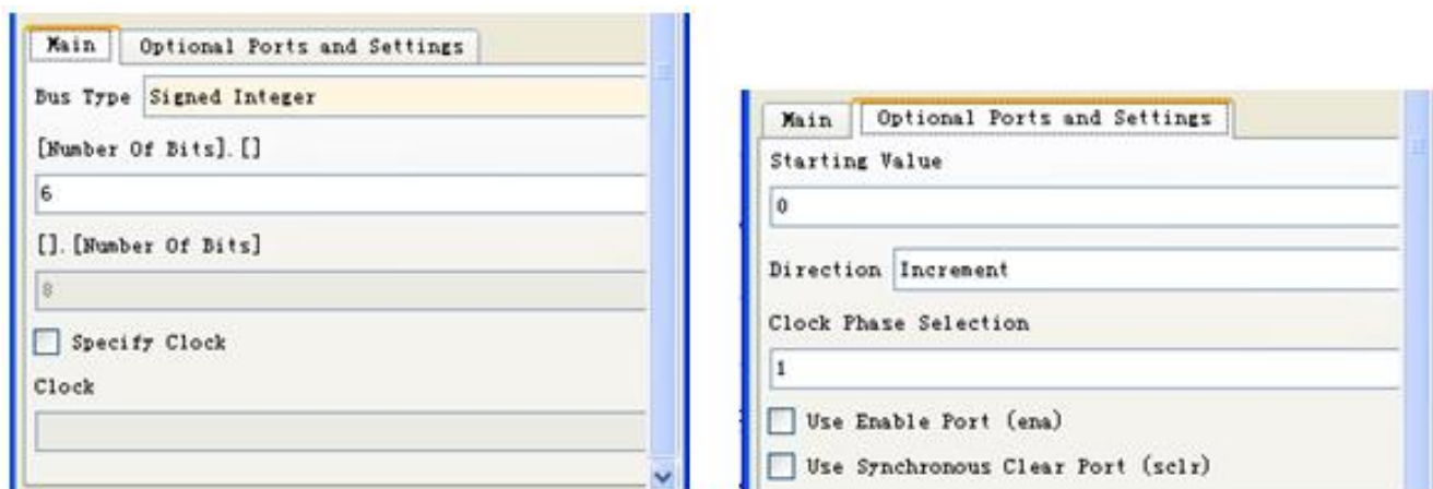
图 11-9 设置递增递减模块
