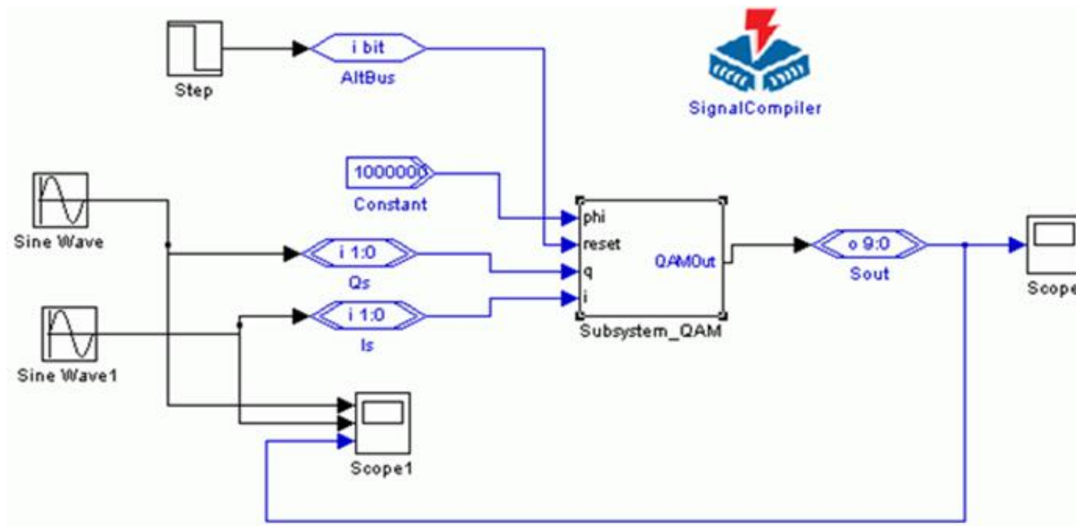
图 11-67 QAM 模型
