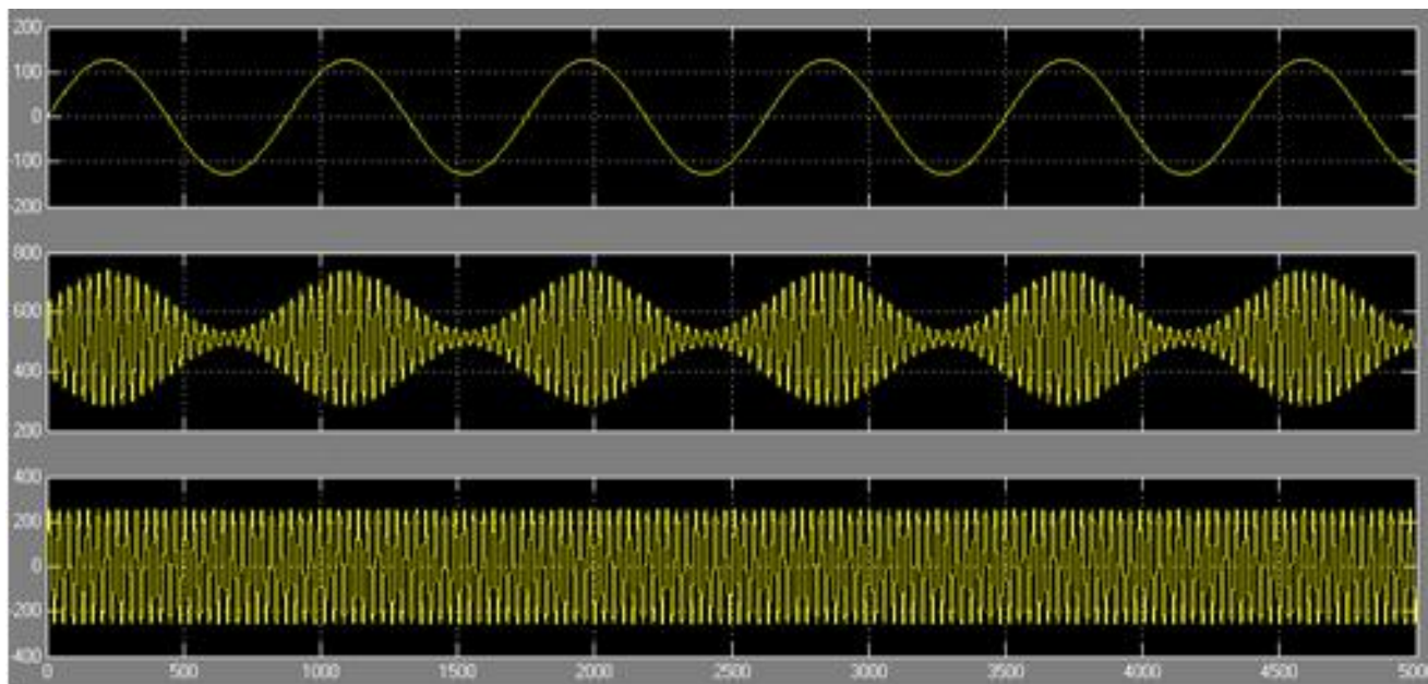
图 11-52 AM 模型仿真波形
