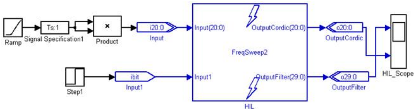
图 11-70 FreqSweep_HIL.mdl 模型电路
