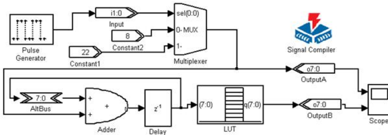
图 11-47 FSK 调制器模型
