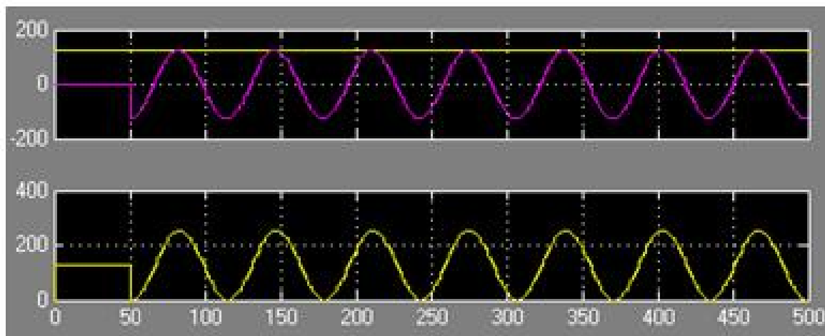
图 11-43 新的 subint 模型的仿真波形图
