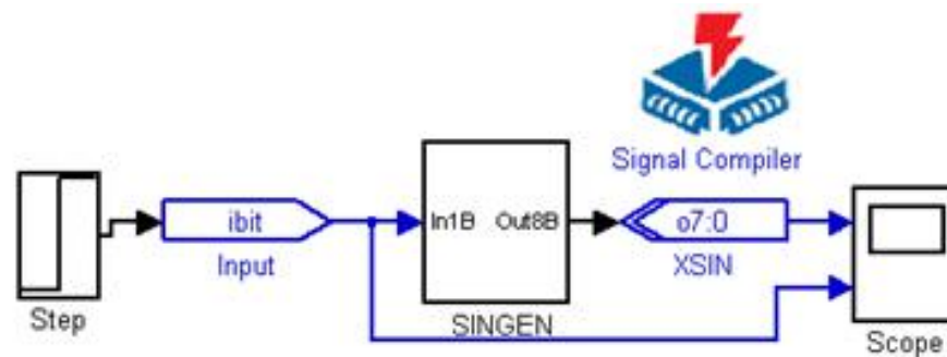
图 11-41 顶层设计图
