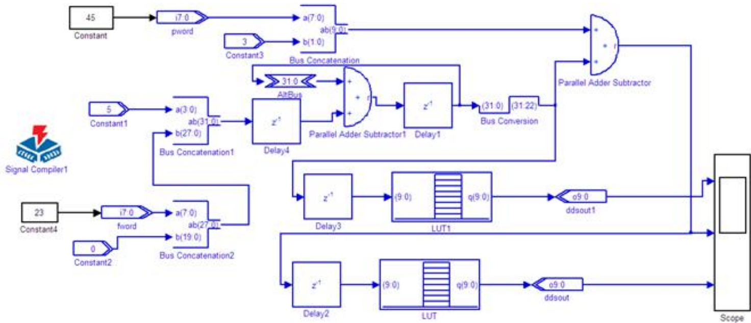
图 11-66 数字移相信号发生器
