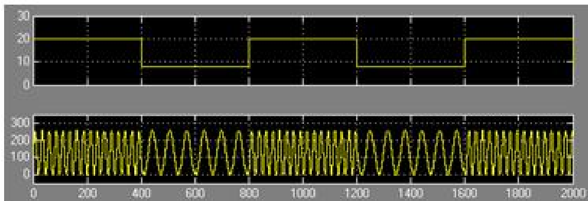
图 11-48 FSK 的 Simulink 仿真结果
