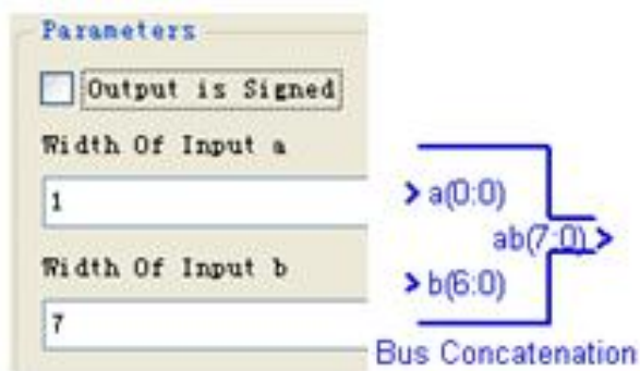
图 11-28 Bus Concatenation 模块设置
