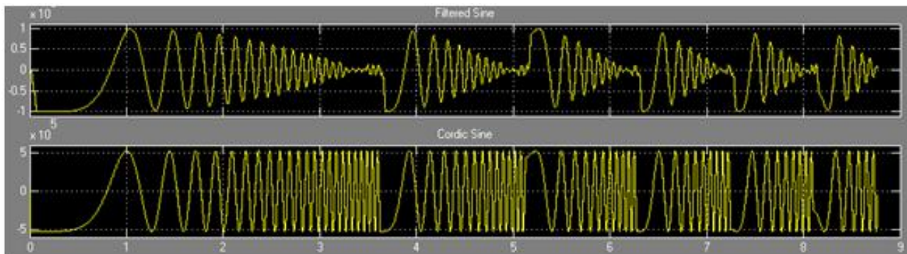
图 11-69 FreqSweep.mdl 模型的 Simulink 仿真波形
